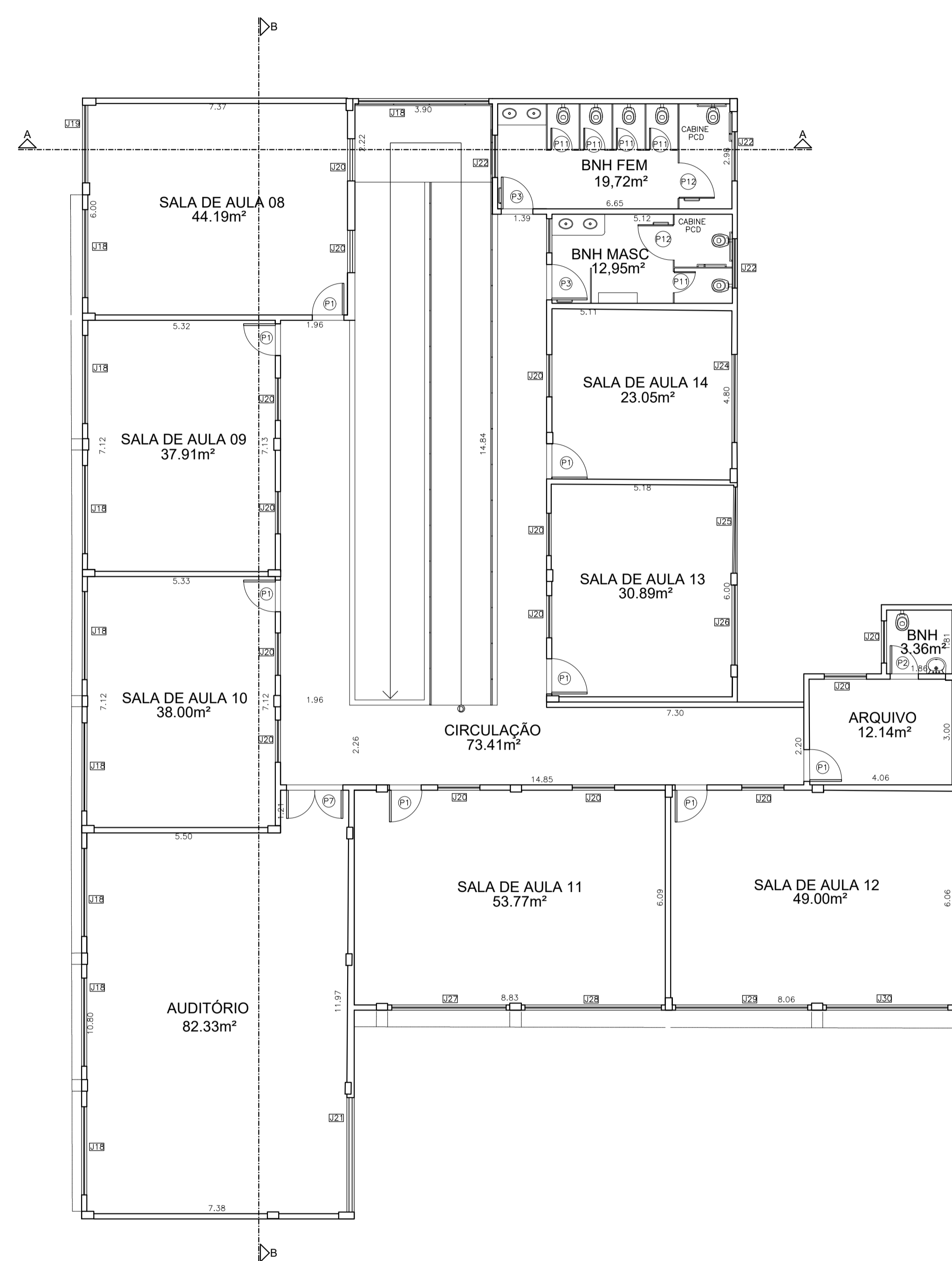
2 PLANTA BAIXA - PAV. SUPERIOR ESCALA 1:100
