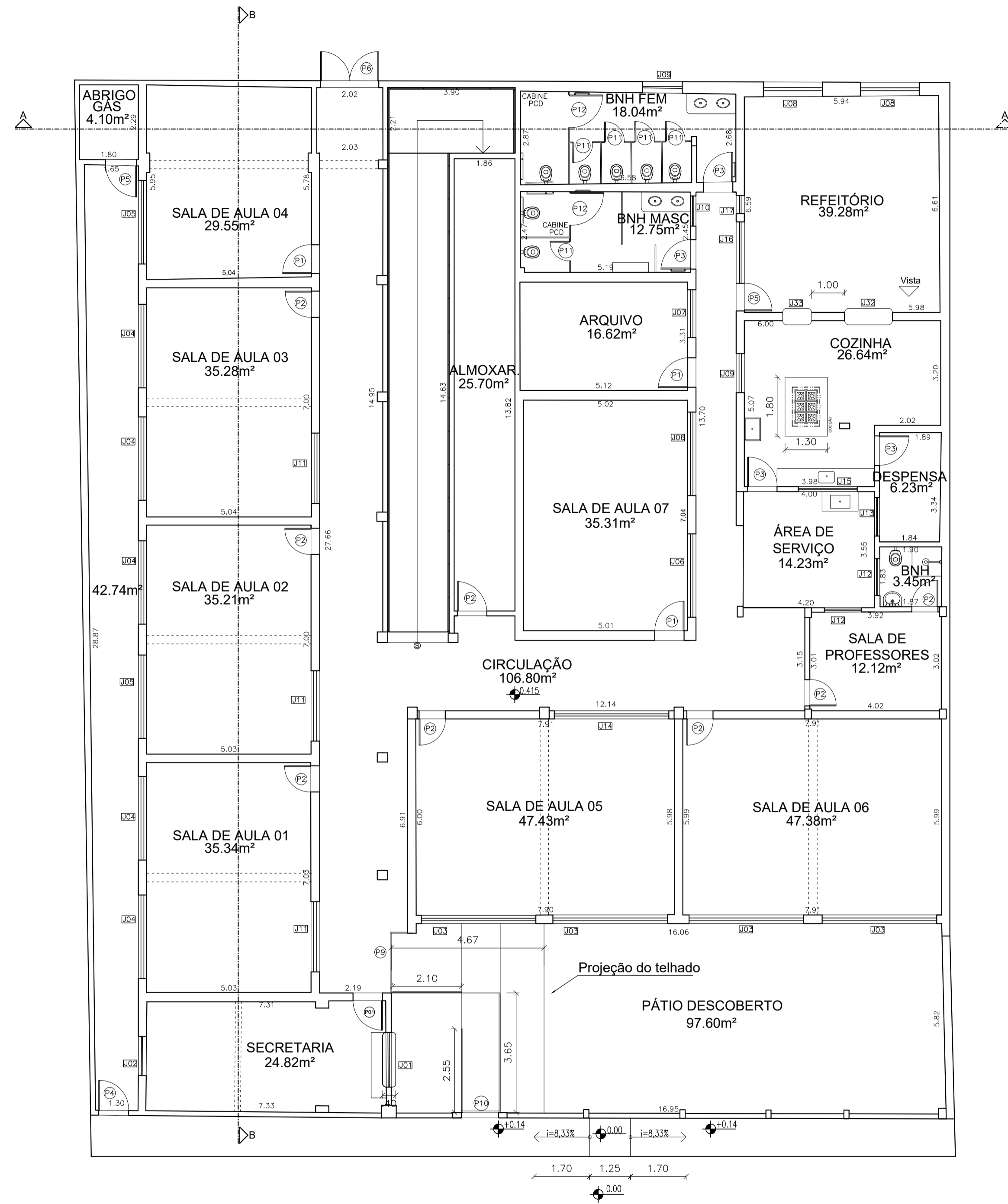
1 PLANTA BAIXA - PAV. TÉRREO ESCALA 1:100
